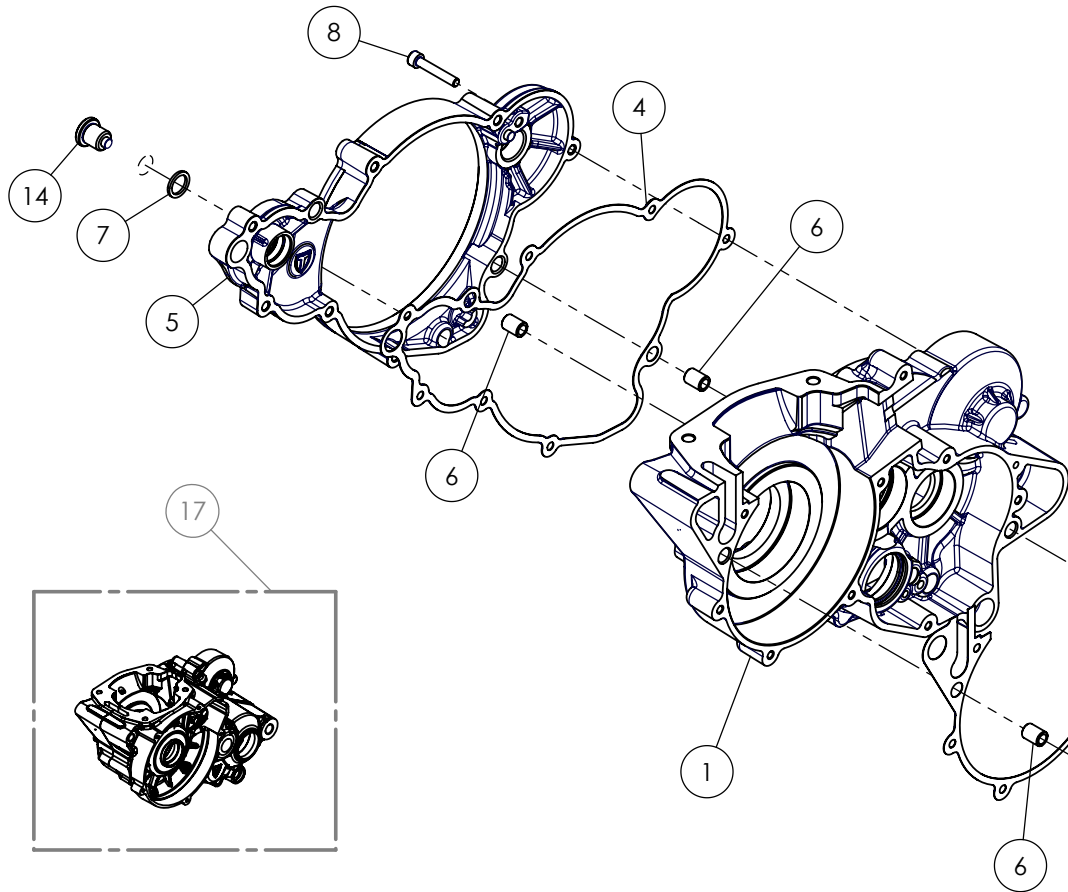
Graphic Engine Longer Bolts - Gráfico Longitud Tornillos
